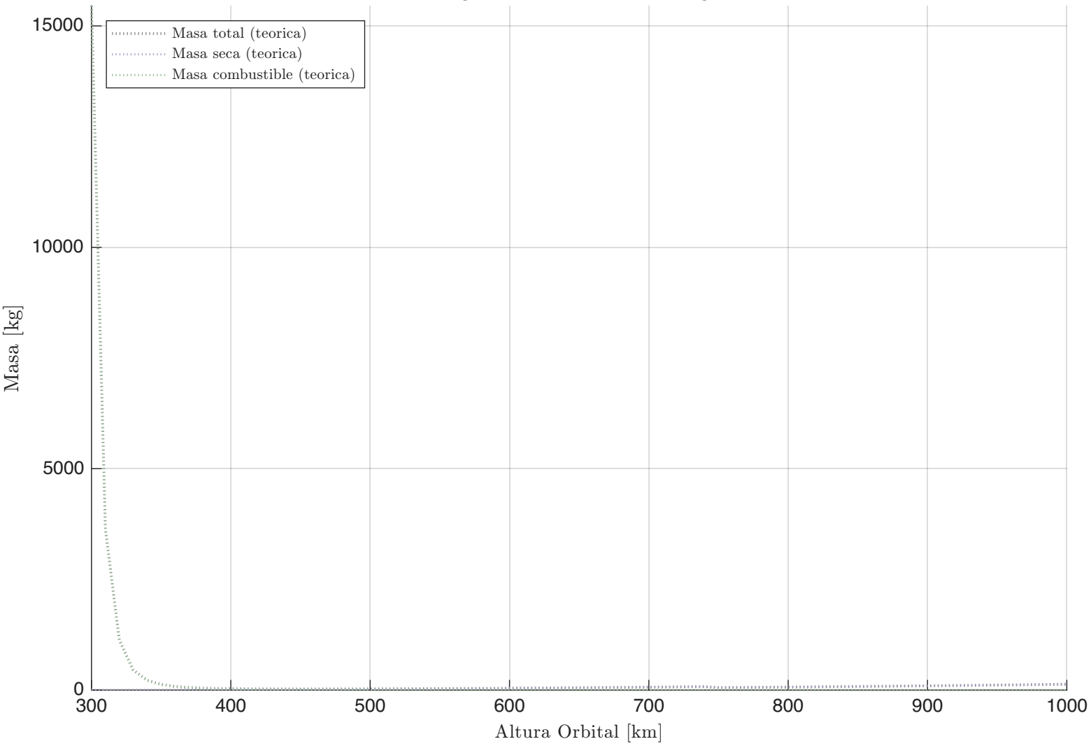
Desglose de Masas vs. Altura Config: 1 Sat, 1 Tel, Det 1, Cassegrain
